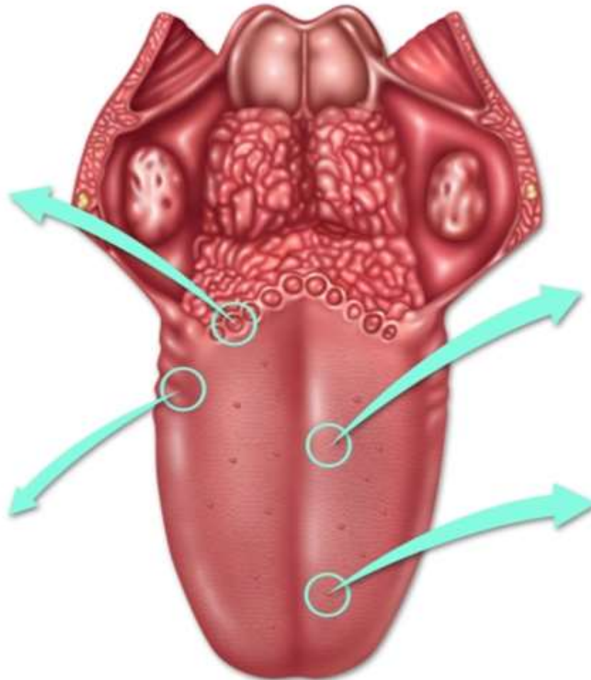
Tongue
